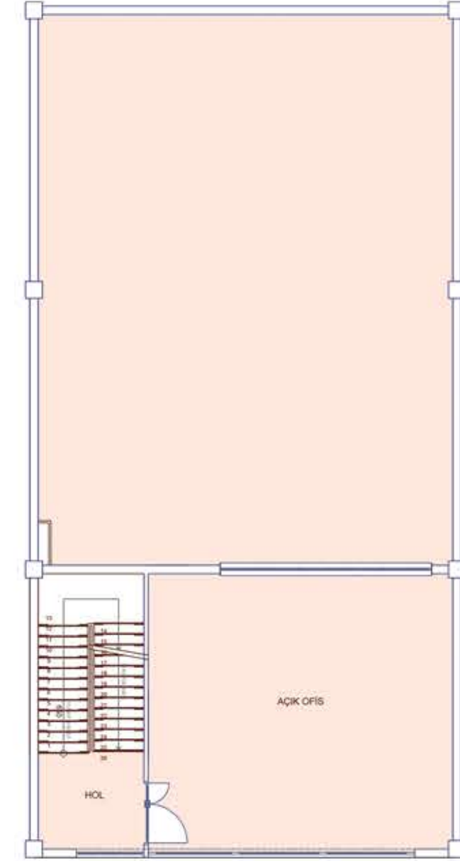
1. Kat Planı
